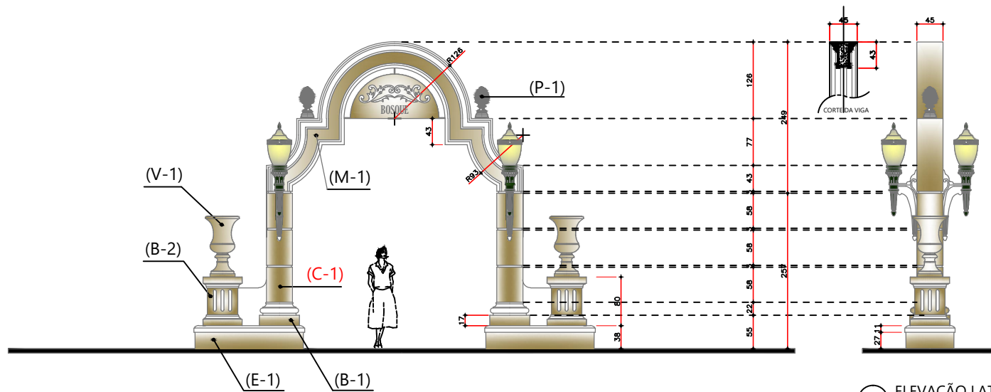
1 ELEVACÃO PRINCIPAL Esc. 1/25
