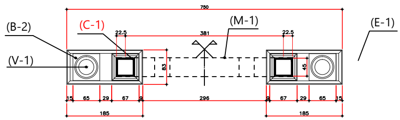
3 PLANTA Esc. 1/25
