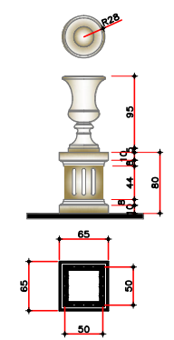
4 VASO Esc. 1/25
