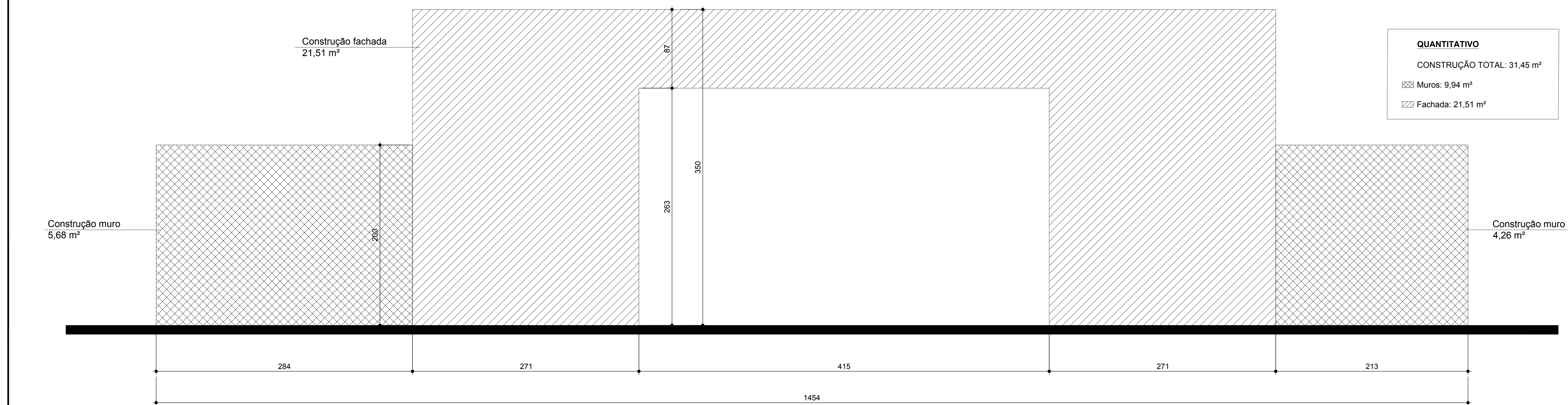
ELEVAÇÃO PÓRTICO 1 | CONSTRUÇÃO
