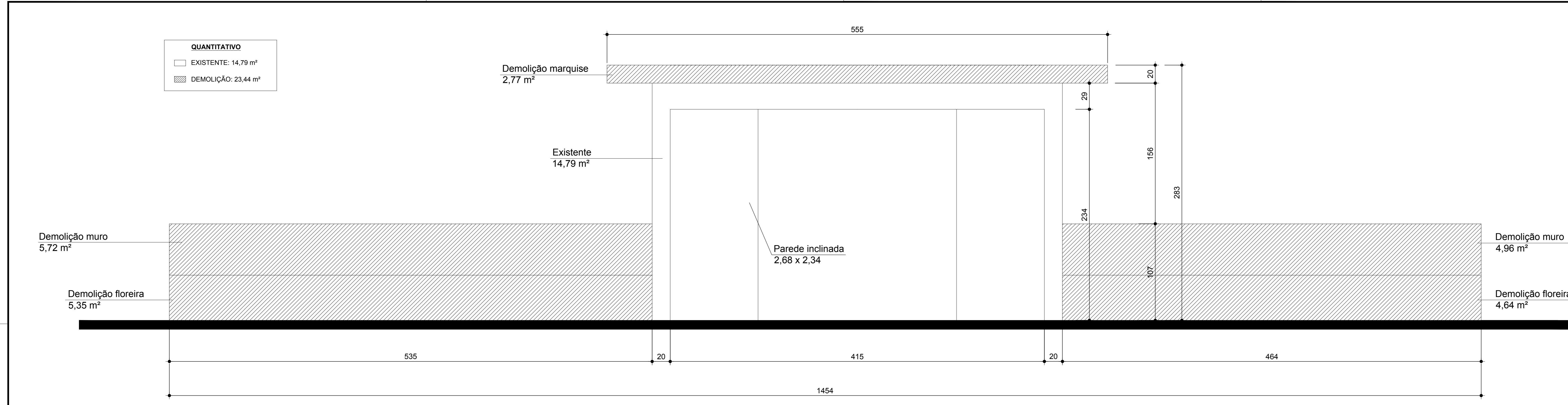
ELEVAÇÃO PÓRTICO 1 | EXISTE E DEMOLIÇÃO
